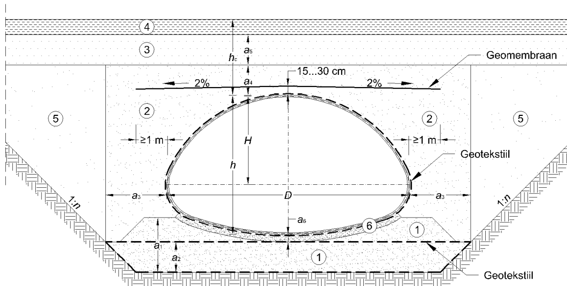
Joonis 15. Pinnase truubi ümber [9]
