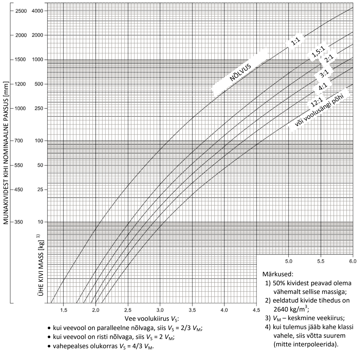
Joonis 17. Kivide kogus lahtise kivilutisega kindlustamisel [31]
