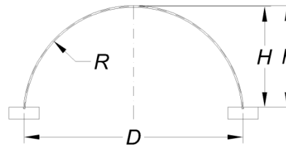
Joonis 7. Terastoruubi tüüp F [9]
