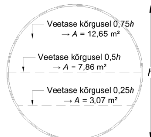
Joonis 10. Näitlik skemaatiline selgitus selle kohta, kui erinevad võivad olla kahe erineva kujuga, kuid sama kõrgusega truupide läbilaskevõime erinevate veetasemete korral
