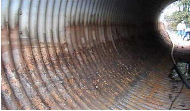
Foto 13. Pöördumatult kahjustatud truubi alaosa [29]
