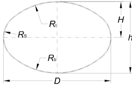
Joonis 3. Terastoruubi tüüp B [9]
