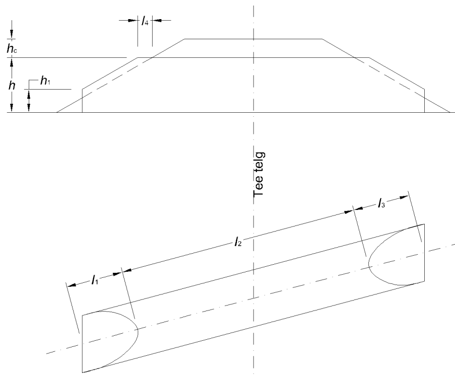
Joonis 12. Truubi pikkuse määramine [12]
